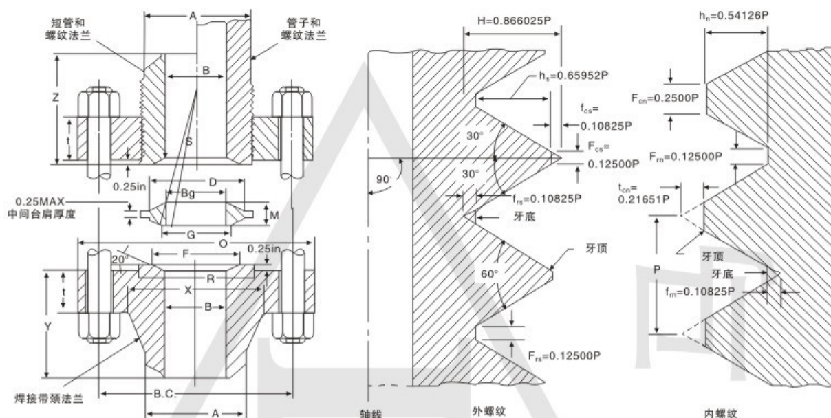
用透镜垫的高压化工法兰和螺纹短管MSS-SP-65 表 4000磅级美标法兰端面加工、透镜垫、法兰和短管的尺寸 (尺寸为mm)
