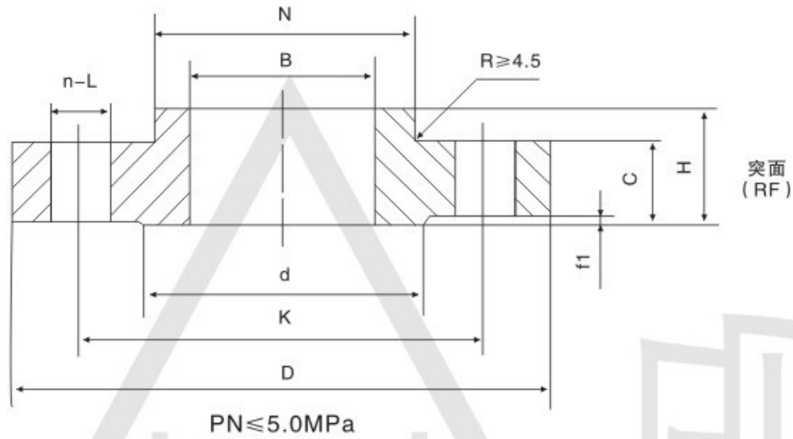
图 美标带颈平焊钢制管法兰 (SO)
