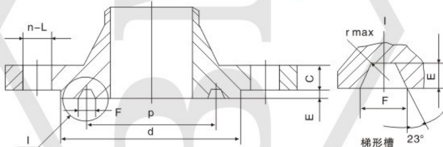
图 美标带颈对焊钢制管法兰(WN) ASME B16.5-2009 HG/T20617-2009
