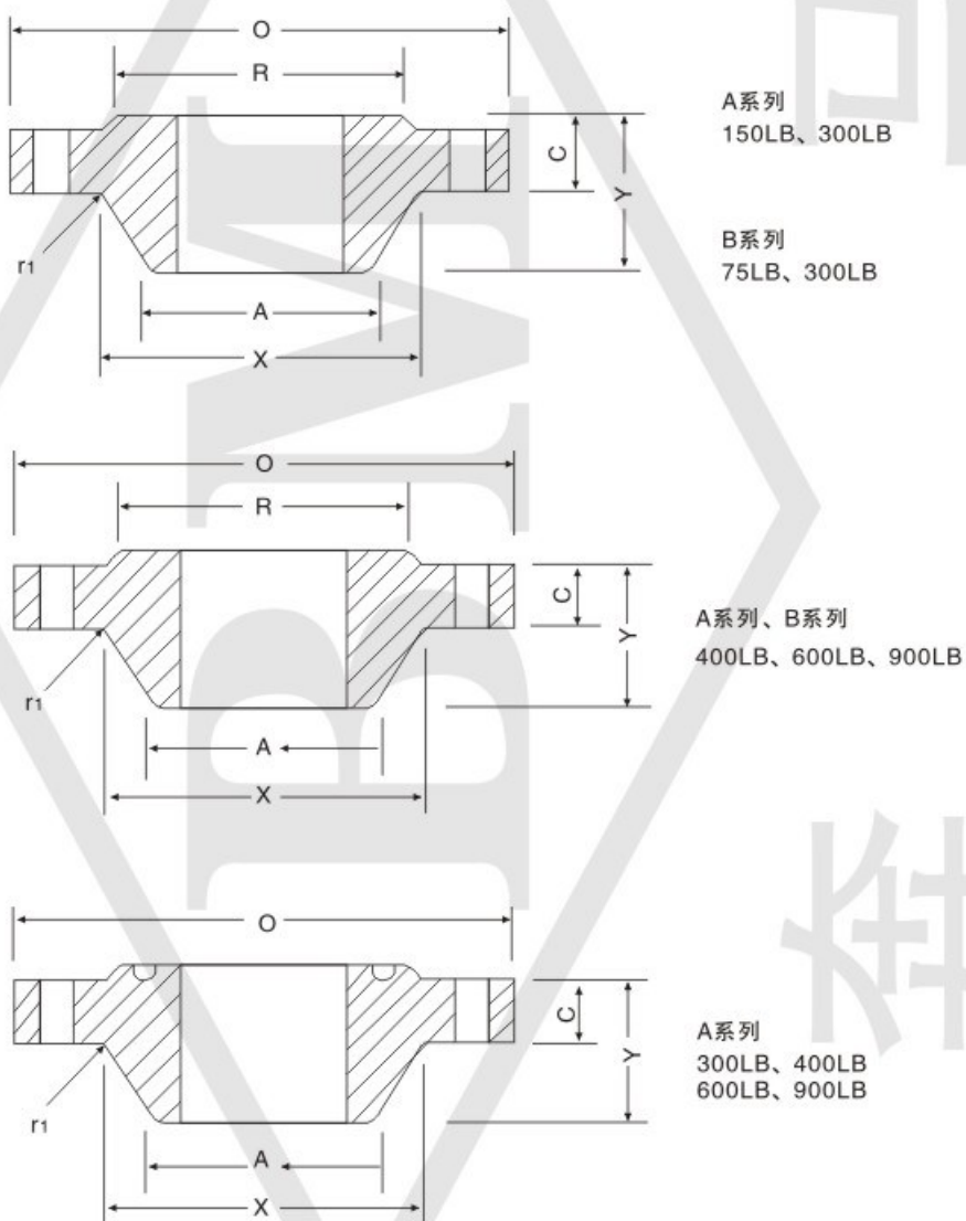
图 美标大直径管钢制法兰 ASME B16.47-2006
