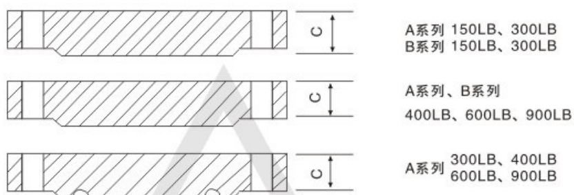
图 美标大直径管钢制法兰盖
